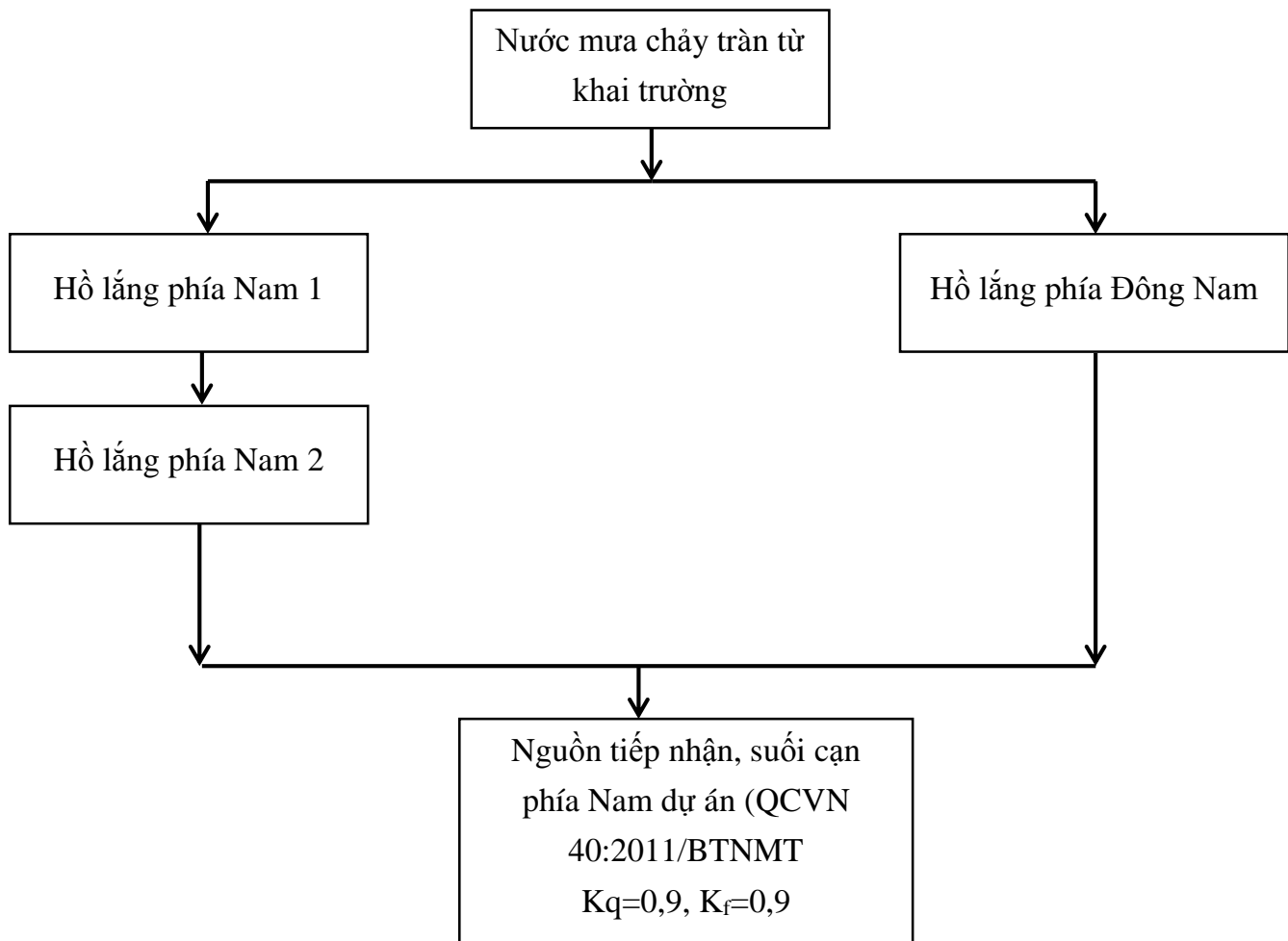
Hình 4.1 : Sơ đồ thu gom nước thải
