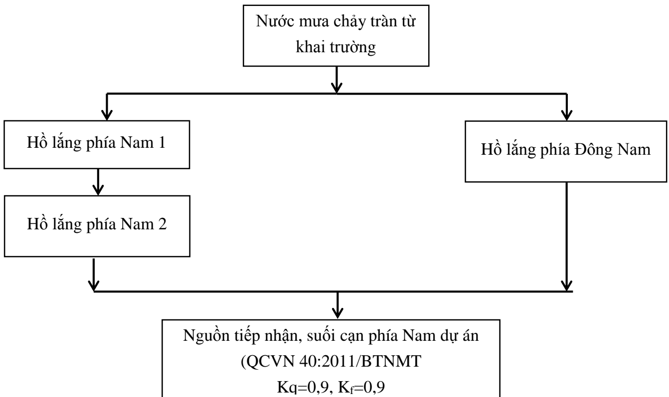
Hình 3.1: Sơ đồ thu gom nước thải
